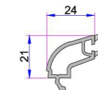
Üçlü Cam Çıtası (32mm) P.A.750.4204.600.0.HC
