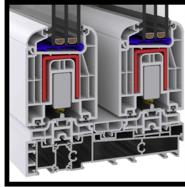
Hebeschiebe Orta Kanal Kapama P.A.930.6505.600
