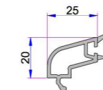
Üçlü Cam Çıtası (32mm) P.A.800.4500.600.0.HC
