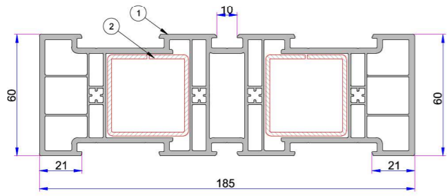
1. Hebeschiebe Kasa Profili P.A.930.1000.600.0.BC.01 2. Destek Sacı (40x40) 2 mm - 34022 - 20110
