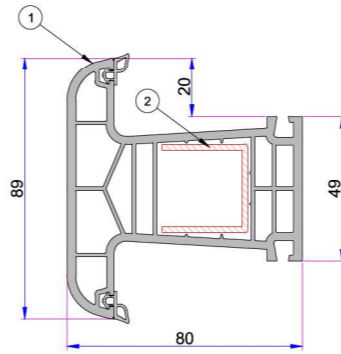
1. Hebeschiebe Orta Kayıt Profili P.A.860.3000.600.0.BC.01 2. Destek Sacı (29x30x29) 1,5 mm - 34022 - 15002 2,0 mm - 34022 - 20002
