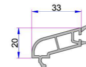
Çift Cam Çıtası (24mm) P.A.800.4200.600.0.HC
