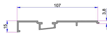
Hebeschiebe Alüminyum Eşik İkinci Kanat Ray (Yeni Yapılacak)
