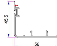
PVC Kanal Arka Bindirme Contası P.A.232.5700.600.0.00.01
