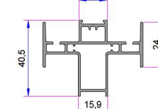
Alm. Kulaklı Çift Kanal Adaptörü AD 16-058
