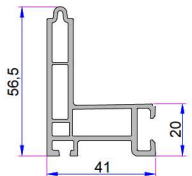
Sineklik Ray Profili P.A.232.5802.600.0.00.19
