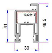
Sürme Sineklik Kanal Profili P.A.242.2305.600.0.00.01
