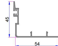
Alm. Kanal Arka Kapama 16051.601.5.1.1.9016
