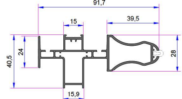
Alm. Griyaylı Çift Kanal Adaptörü AD 16-059
