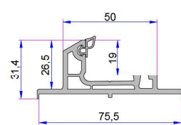
Çift Ray Adaptör Profili P.A.232.5800.600.0.00.19
