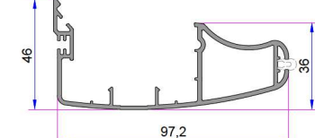
Alm. Kanal Arka Kapama Griyay Profili AD 16-061
