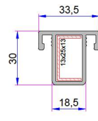
Sürme Sineklik Orta Kayıt Profili P.A.242.3200.600.0.00.01
