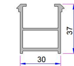
Kasa Montaj Profili P.A.060.5301.600.0.00.19
