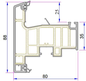
Dışa Açılım Kanat Profili P.A.883.2001.2
