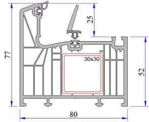
Süper Kasa Profili P.A.888.1001 Destek Sacı (30x30)
