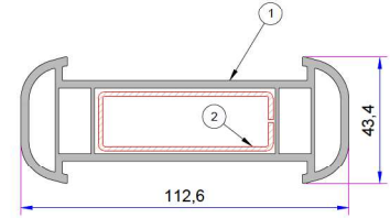
1. Kalın Bağ Profili P.A.080.5000.600.0.00.19 2. Destek Sacı (20x60) 1,2mm - 34022 - 12106 1,5mm - 34022 - 15106 2 mm - 34022 - 20106
