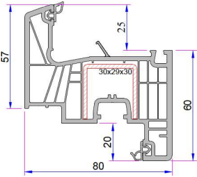
Kanat Profili P.A.888.2000 Destek Sacı (30x29x30)
