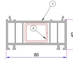
1. Kasa Yükseltme Profili P.A.080.5300.600.0.00.19 2. Destek Sacı (30x25) 1,2mm - 34022 - 12119 1,5mm - 34022 - 15119 2 mm - 34022 - 20119
