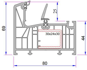
Kasa Profili P.A.888.1000 Destek Sacı (30x24x30)
