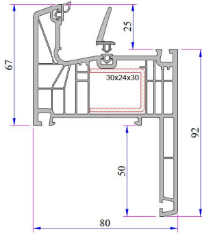
Pervazlı Kasa Profili P.A.888.1200 Destek Sacı (30x24x30)
