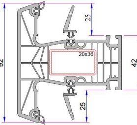
Orta Kayıt Profili P.A.888.3000 Destek Sacı (20x36)
