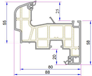
Damlalıklı Kanat Profili P.A.883.2200.2
